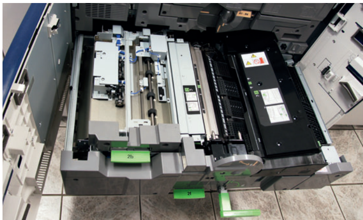
Das gut zugängliche Innenleben der Xerox Versant 2100 Press ist Garant für schnellen Farbtonerwechsel und fix erledigte Service-Einsätze.
